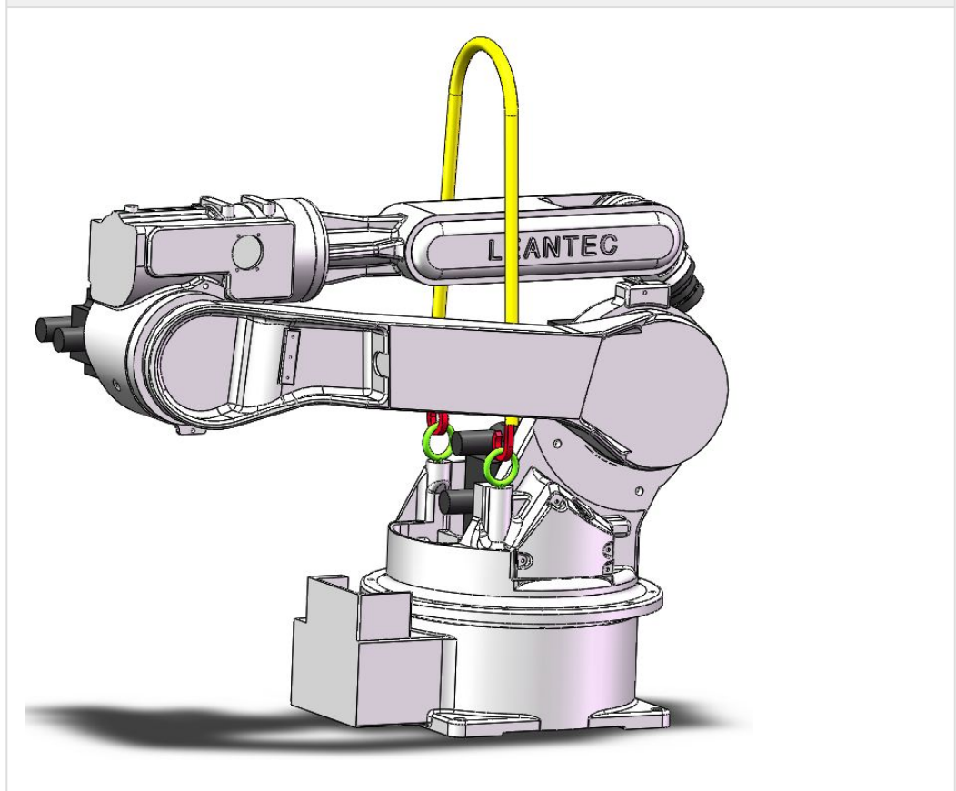
LA1717-20机器人本体出厂姿态及吊装方式示意图
